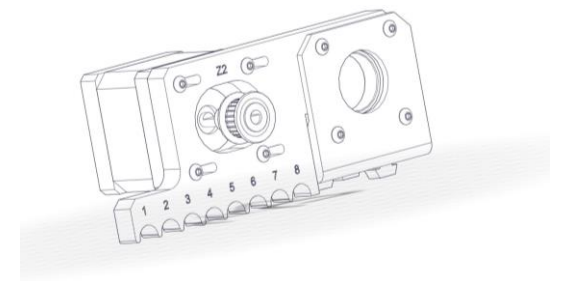
Z2 brackets
